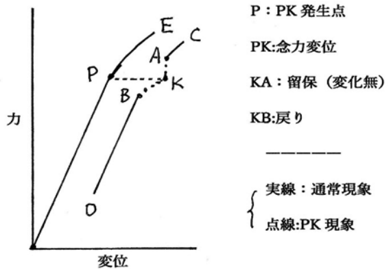
図2 PKの進行方向に働く戻し作用
